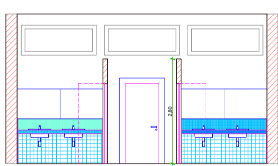
Sezione servizi igienici lato ovest
