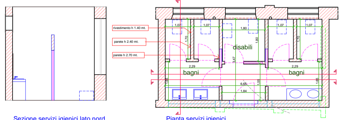
Pianta servizi igienici
